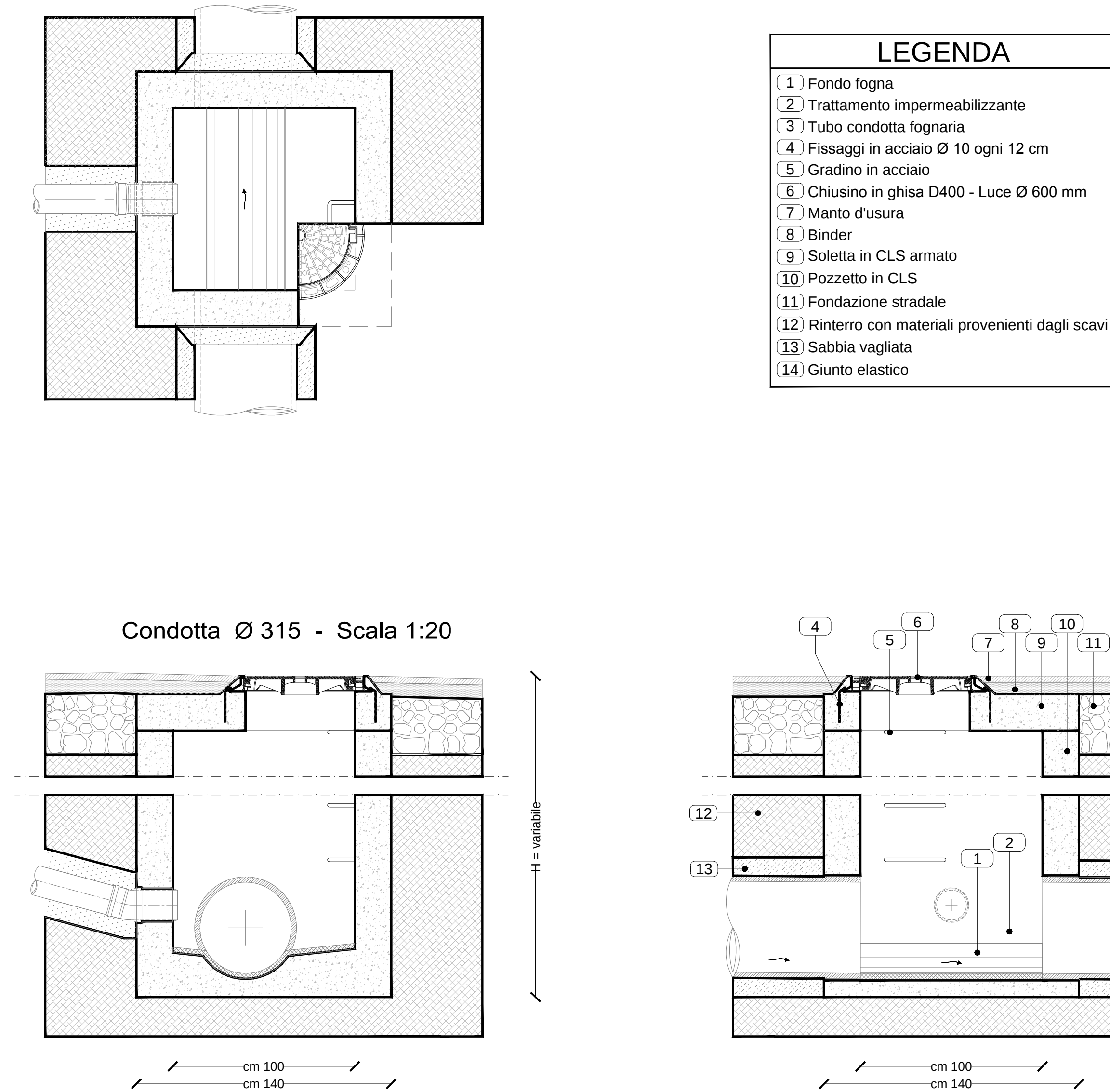
POZZETTO ISPEZIONE IN LINEA - Immissione caditoia
