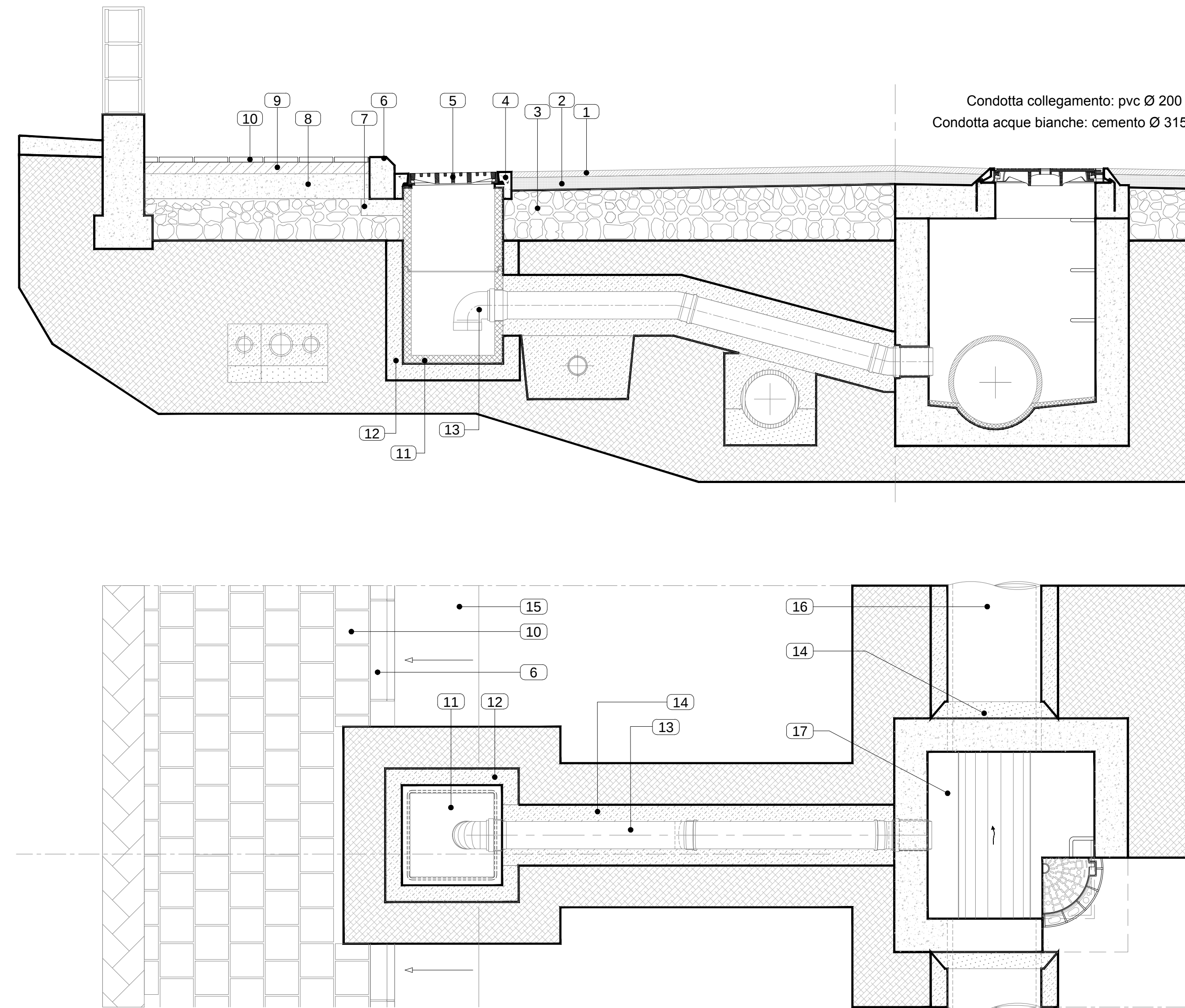
COLLEGAMENTO CADITOIA - pozzetto - Scala 1:20
