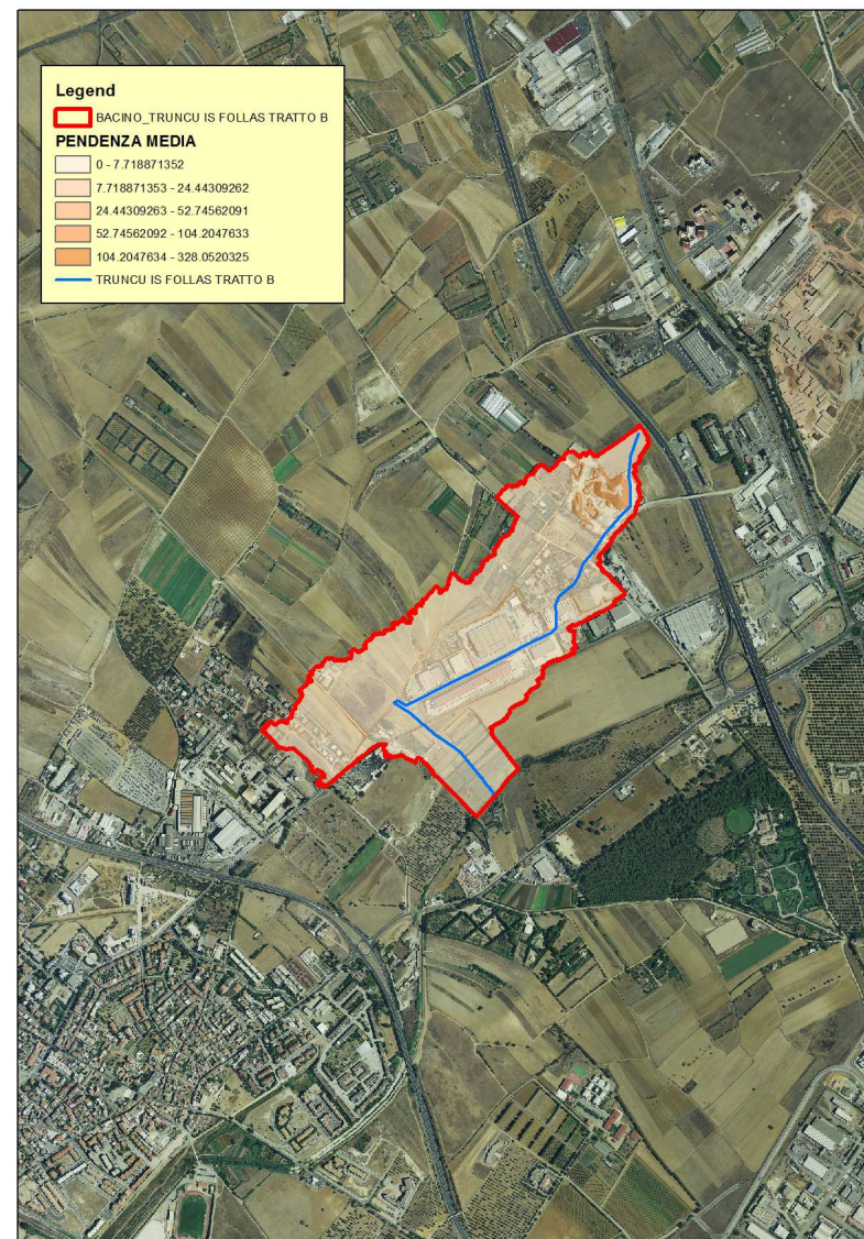
Figura 5 Pendenza media Bacino
