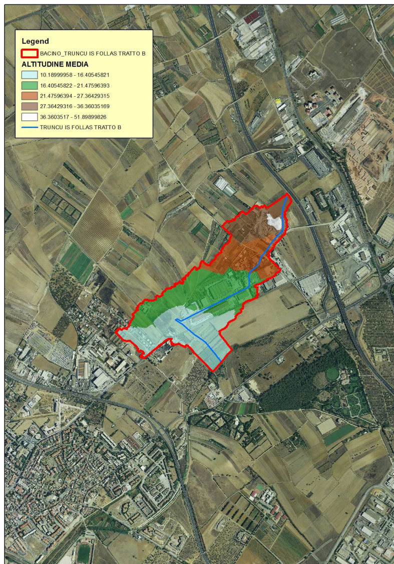
Figura 4 Altitudine media Bacino
