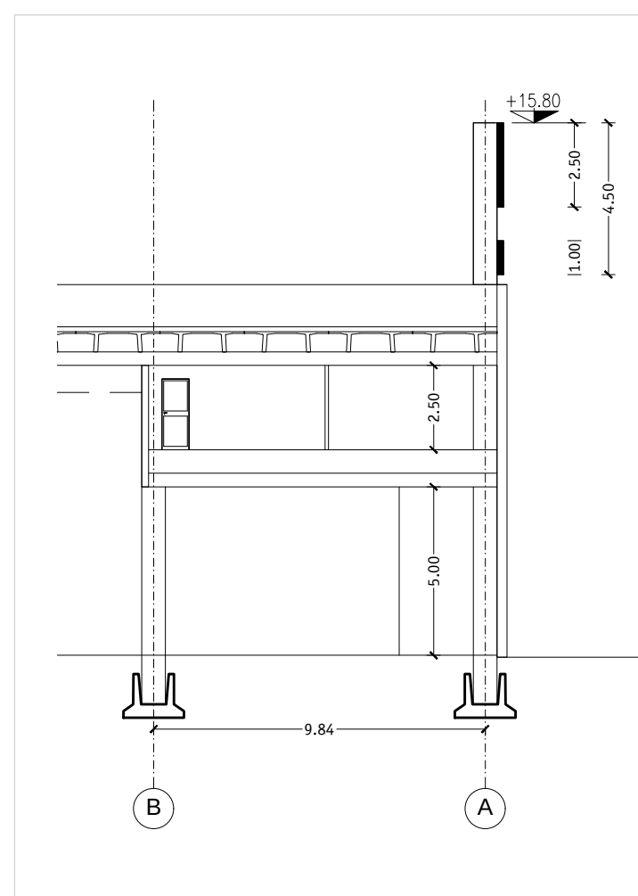
SEZIONE A-A SCALA 1:200
